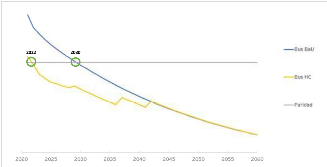
Figura N° 31 - Paridad TCO del escenario Business as Usual y High Case para buses de 12 metros
