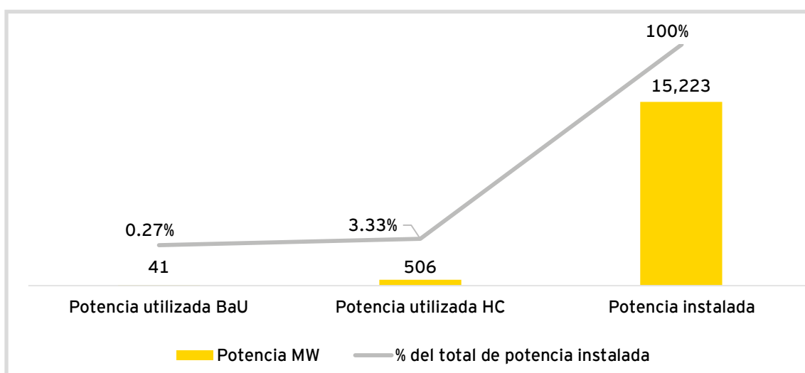
Figura N° 46 - Potencia utilizada por el parque automotor enchufable del año 2030 (MW)
