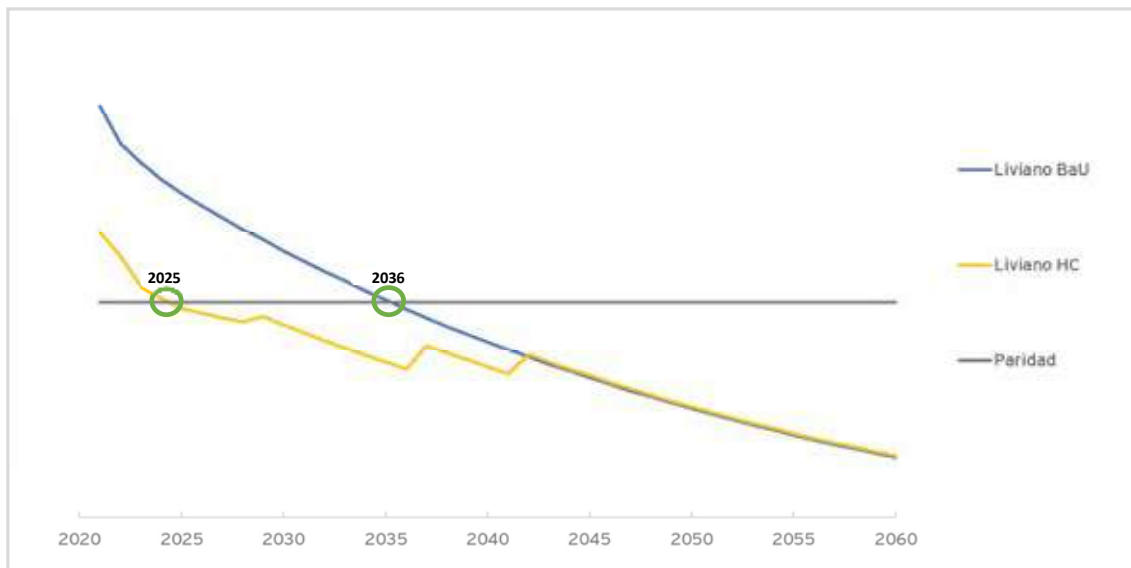
Figura N° 30 - Paridad TCO del escenario Business as Usual y High Case para vehículos livianos (sedán más vendidos)
