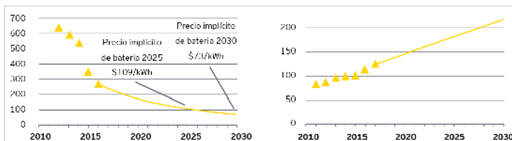
Figura N° 9 - Precio de baterías de EV de Li-ion y peso promedio de la densidad energética histórica y pronosticada
