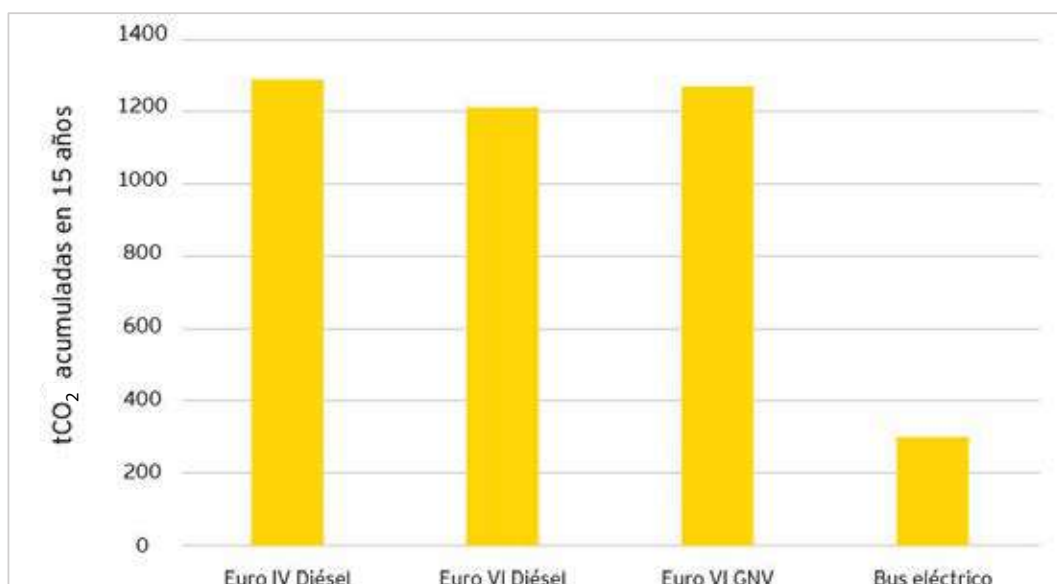
Figura N° 27 - Toneladas de CO 2 eq acumuladas en 15 años para un bus de 12 metros
