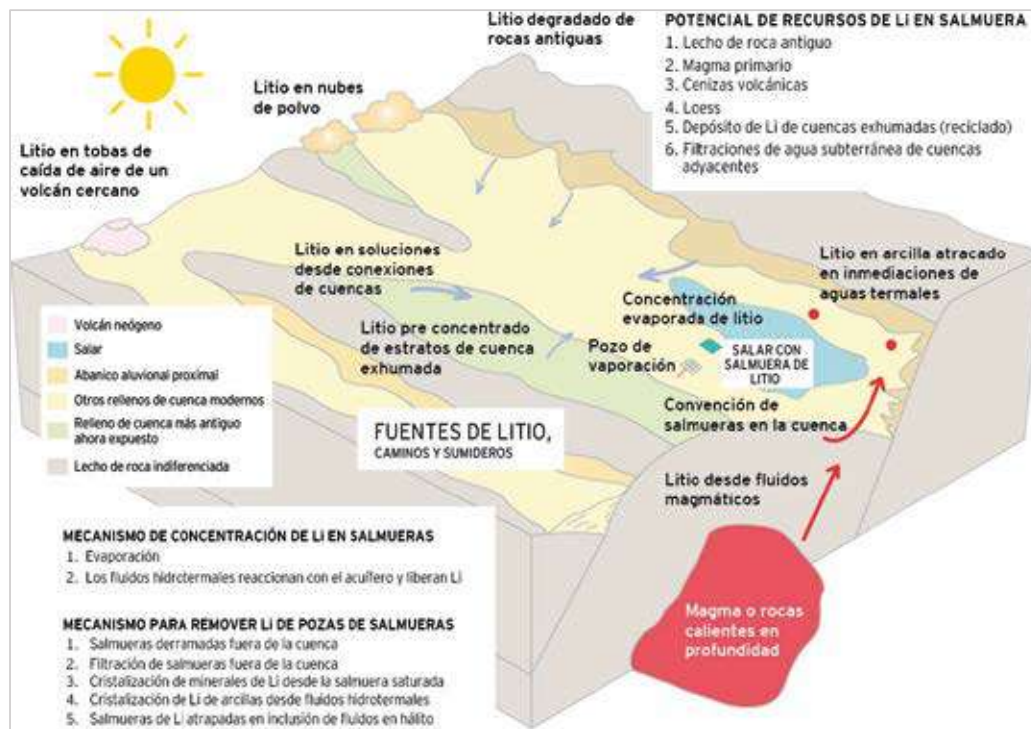
Figura N° 22 - Modelo de depósito para salmuera de litio
