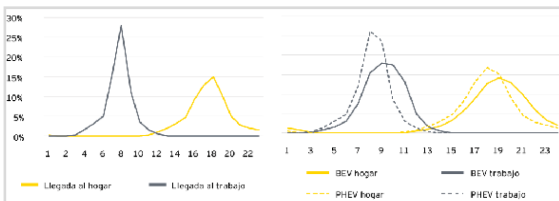
Figura N° 43 – Perfil de consumo y carga en Alemania (% de consumo durante el día)
