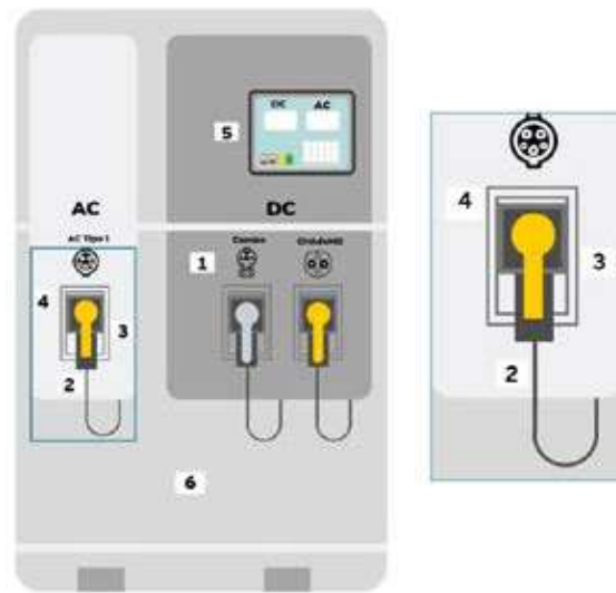
Figura N° 2 – Componentes de una estación de carga semi-rápida y rápida
